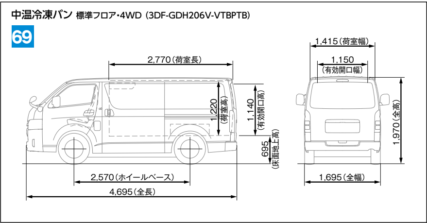
寸法図 (単位:mm)
